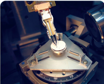
↑ Chronogrip, Mikrogreifer für Miniaturobjekte ©Percipio Robotics
